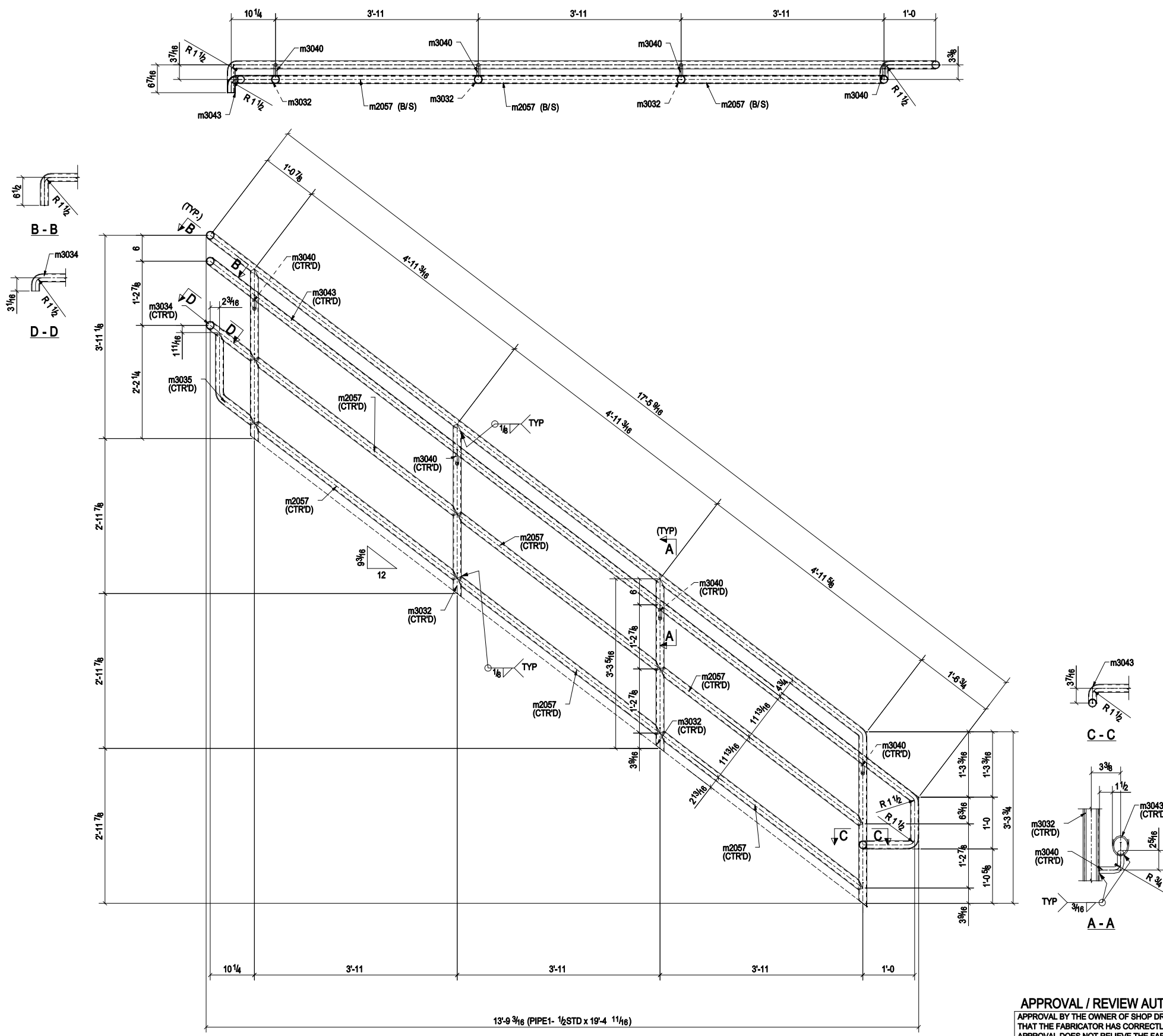
ONE - HANDRAIL - 3832A (GALV.)
